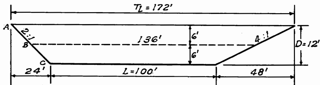
LONGITUDINAL SECTION
