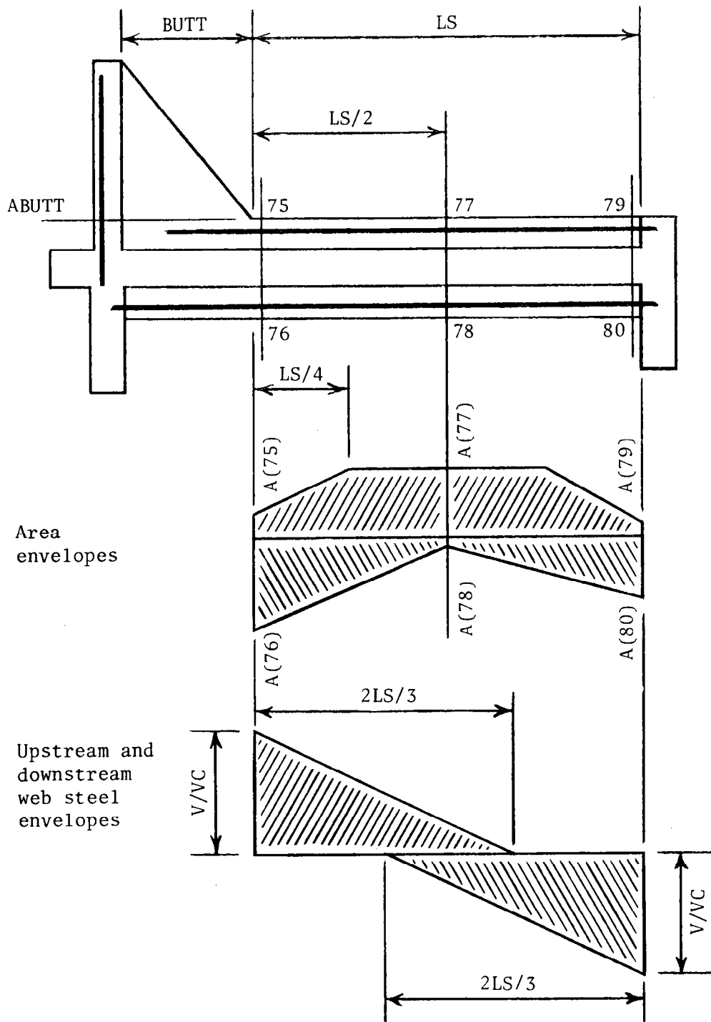
Figure 43. Longitudinal sill steel.
