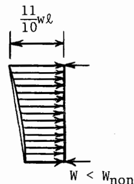
(d) longitudinal sill loading with yielding transverse sill
